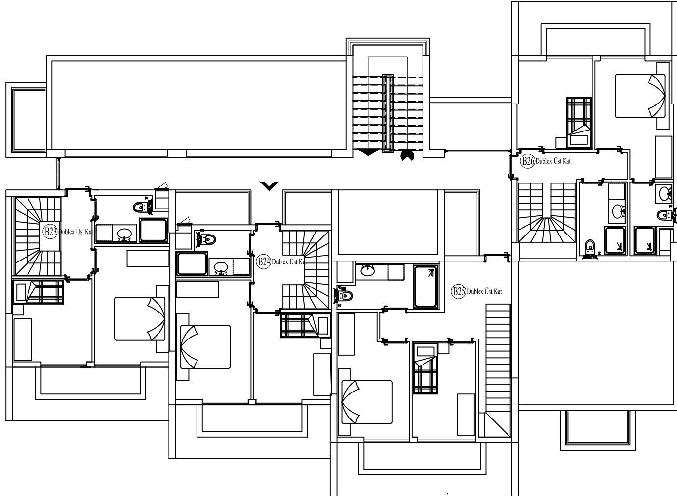
B BLOK ÇATI KATI PLANI ÖLÇEK :1/50 B BLOK : ±0.00=139.50
